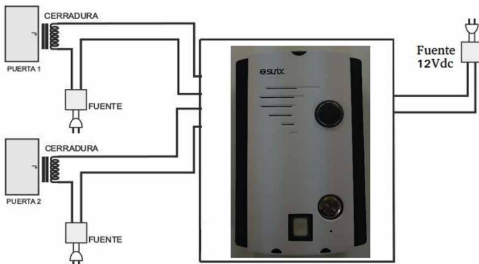
Figura 5 – Conexión general del IP Access
