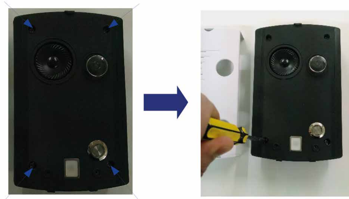
Figura 3 – Desarme de IP Access
