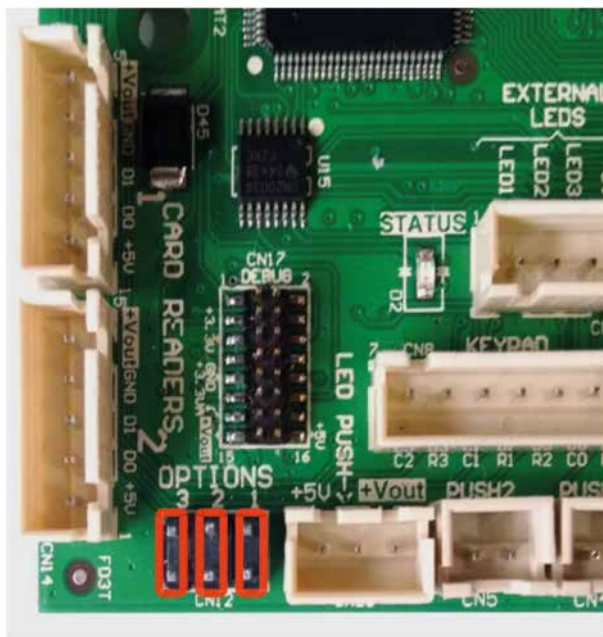
Figura 11 – Pines de configuración para forzar al equipo a los valores de fábrica.
