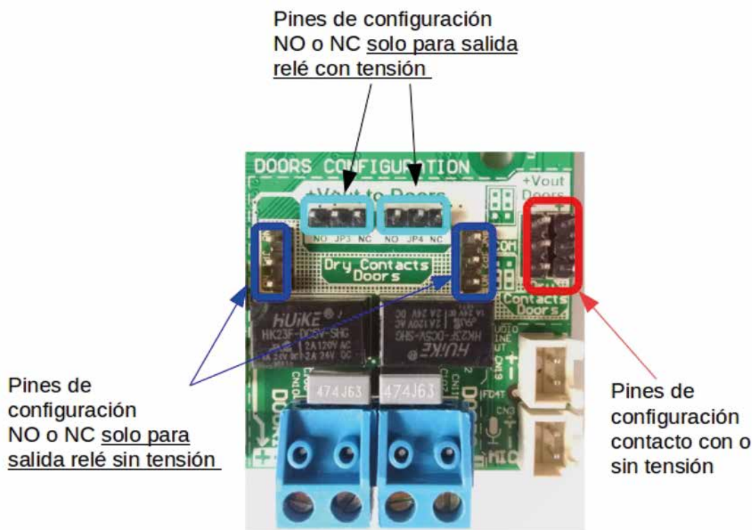
Figura 9 – Área de pines de configuración de relé
