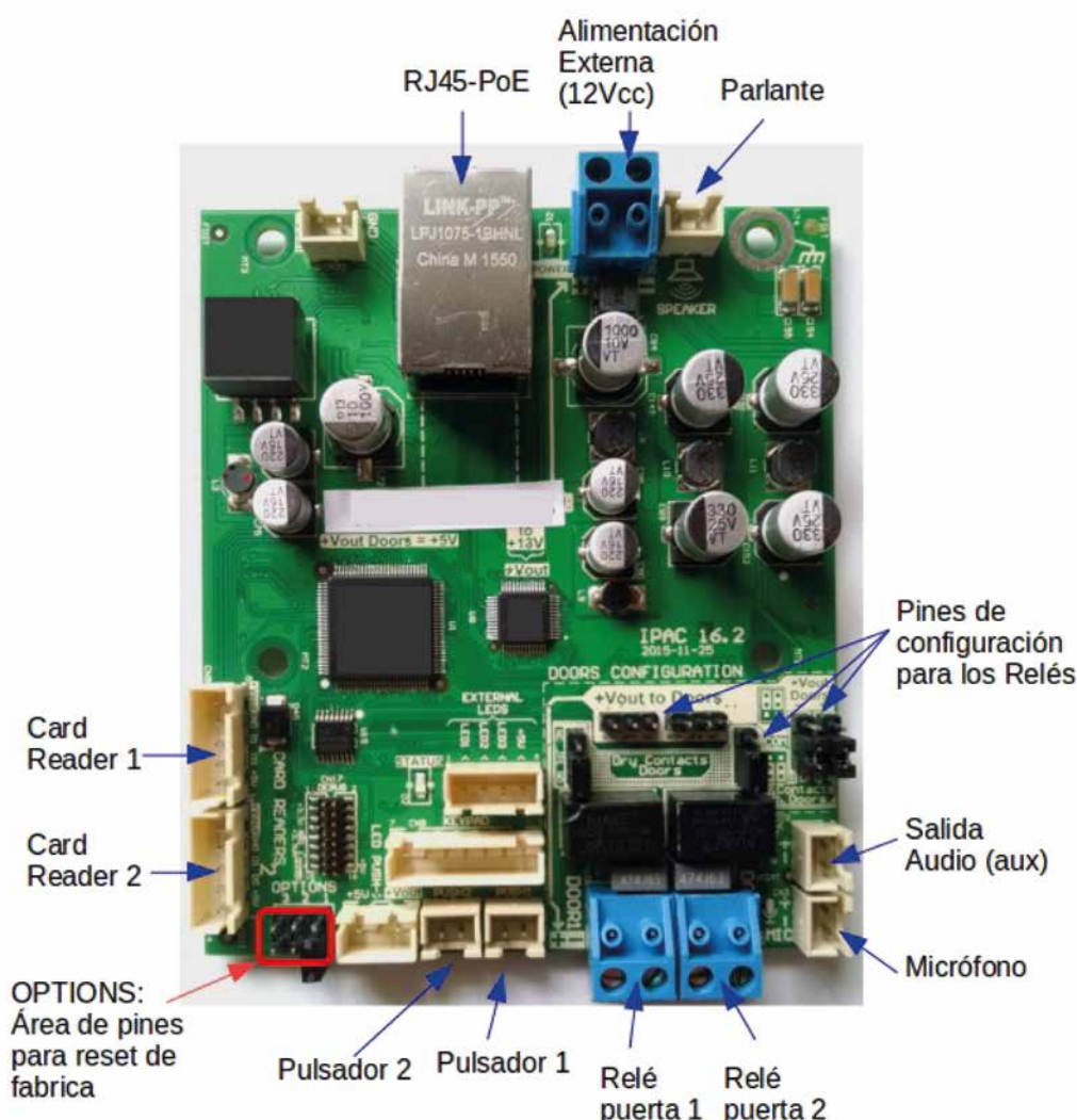
Figura 8 – Placa electrónica de IP Access con videocámara
