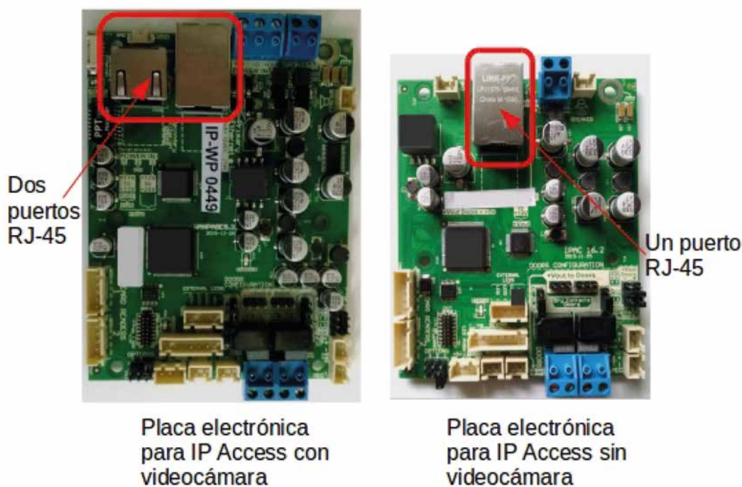
Figura 6 – Modelos de placa electrónica de IP Access
